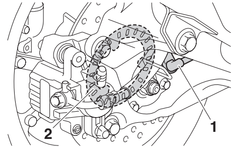
1. 後輪速度感知器 2. 後輪感知器轉子
